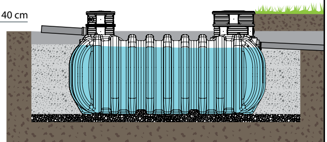
Montage der UNGROUND EXTENSION – Aufsätzen unter schwierigen Bedingungen mit einheimischem Boden und Entlastungsschicht.
